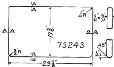
Door Glass No. 75243
